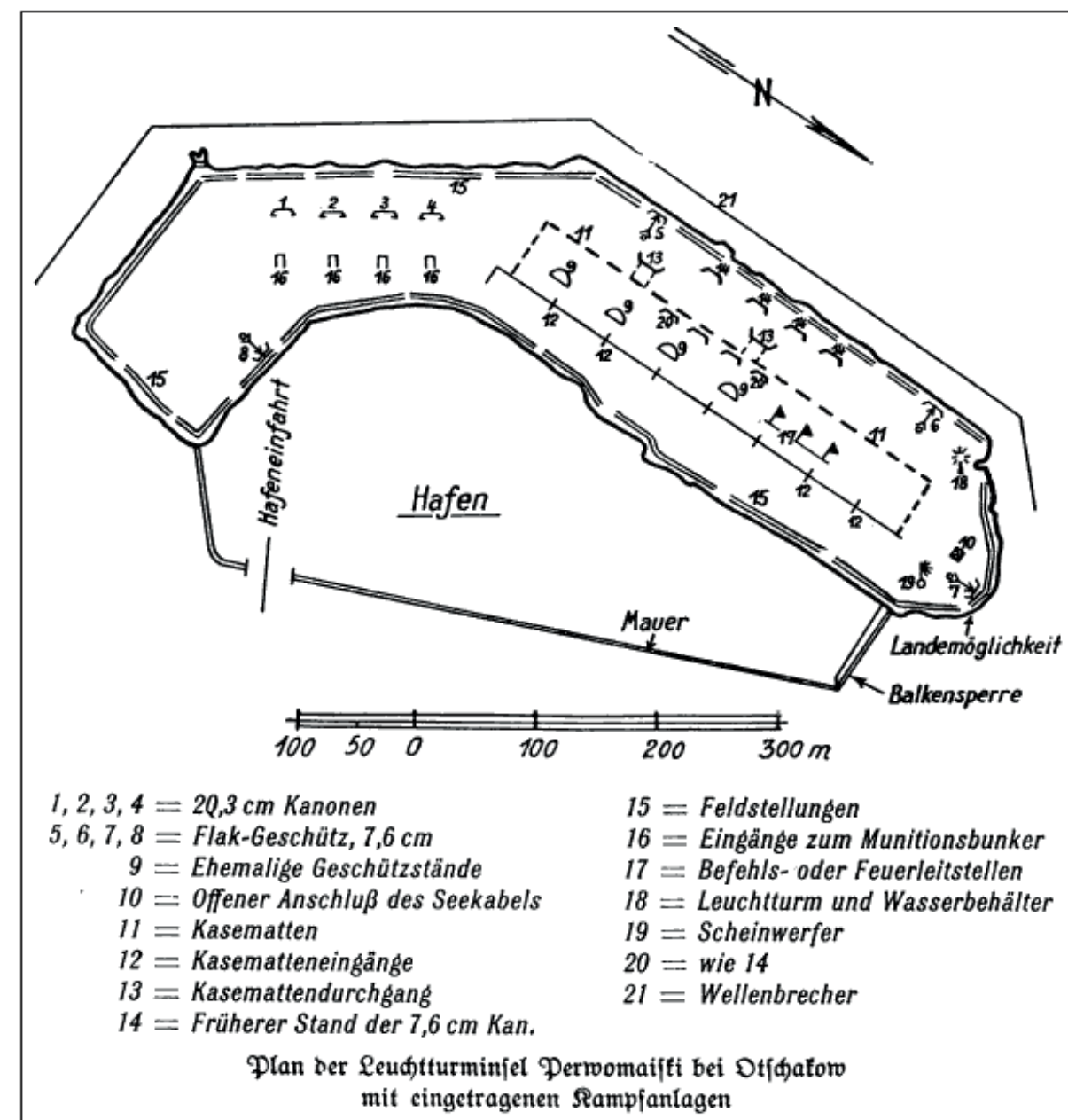
Схема острова Первомайский по состоянию на конец 1941 года выполнена немецкими офицерами. 1,2,3,4 – 203-мм установки; 5,6,7,8 – 76-мм зенитные пушки.
