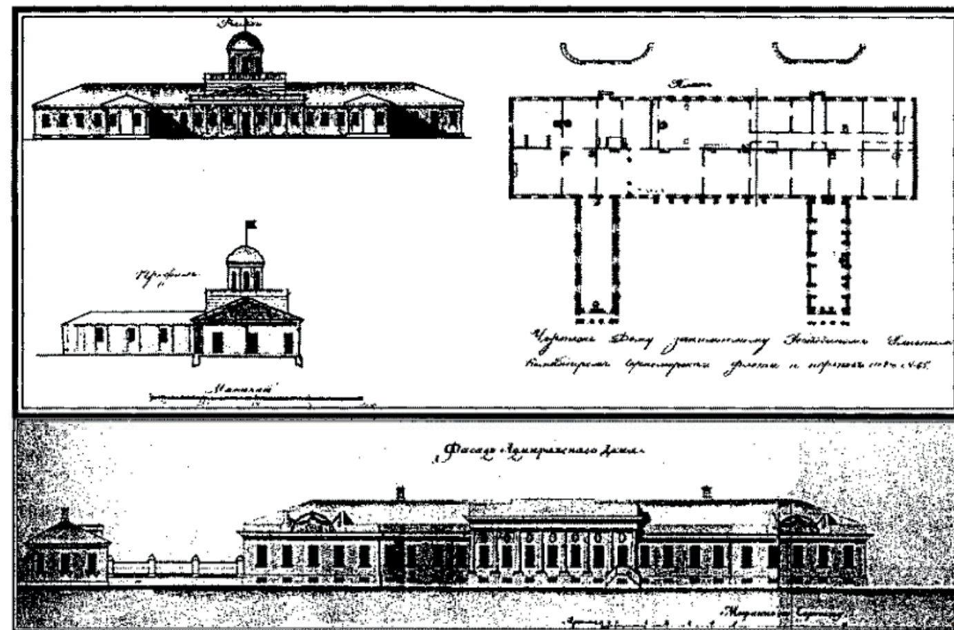
Фасад адмиральского дома. Чертеж 1795 года. Военный инженер И.И.Князев (внизу)
